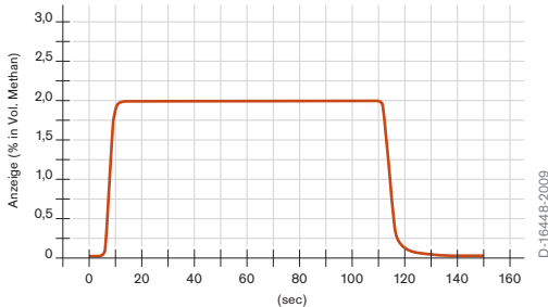
Ansprechzeit des DrägerSensor CatEx 125 Mining PR im X-am 5000
