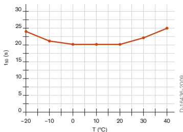
Ansprechzeit (t 90 ) vs. Temperatur begast mit 5000 ppm CO 2
