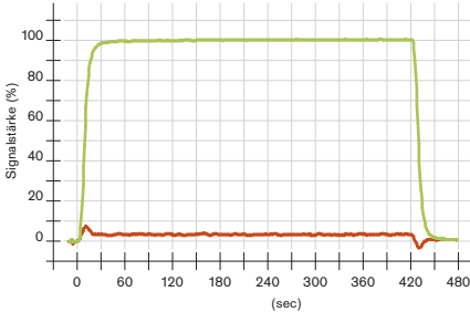
Begastungskurve CO bei 20 °C Flow = 0,5 l/min, begast mit 100 ppm CO
