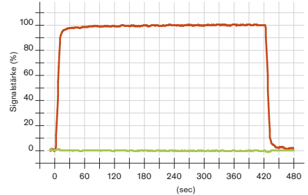
Begastungskurve H 2 S bei 20 °C Flow = 0,5 l/min, begast mit 20 ppm H 2 S
