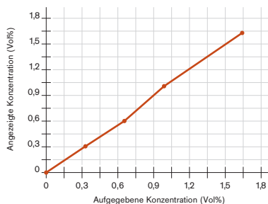
Linearität des XXS H 2 HC Sensors kalibriert mit 1,63 Vol% H 2
